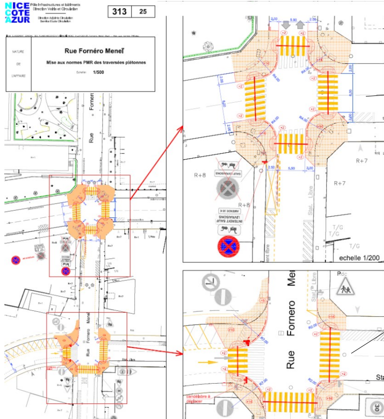
Aménagement des carrefours Rue Fornero Menei - St Roch - Nice
